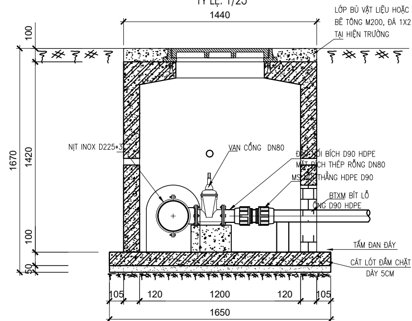
MẶT CẮT 1-1
