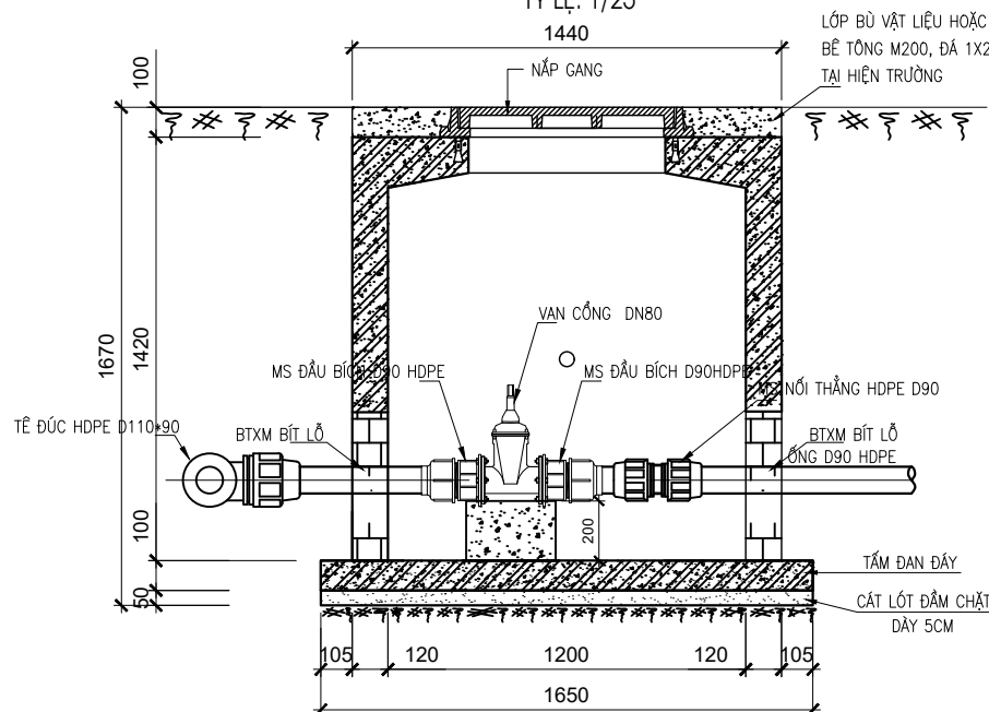
MẶT CẮT 1-1
