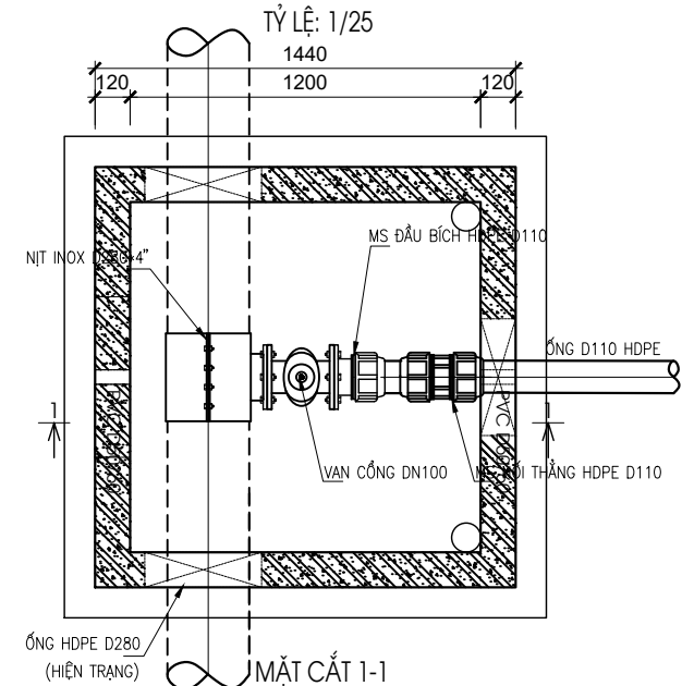
CHI TIẾT KHỞI THỦY ỐNG D110 HDPE VÀO ỐNG HDPE D280
