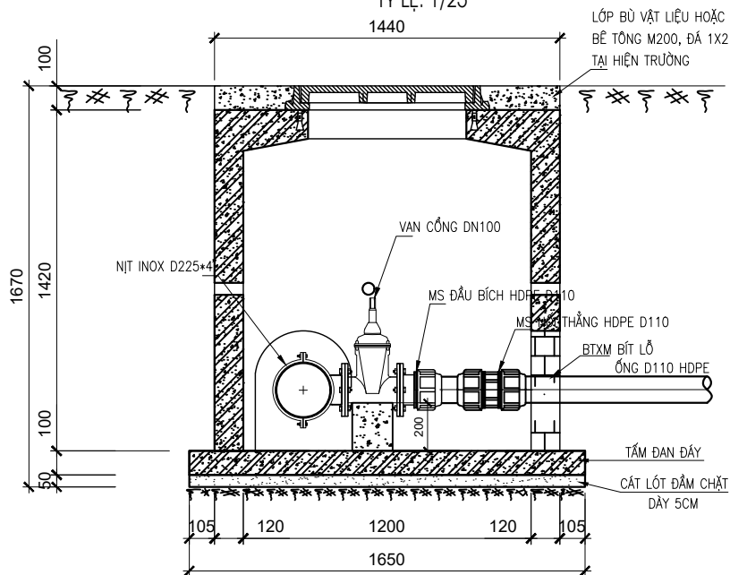
MẶT CẮT 1-1
