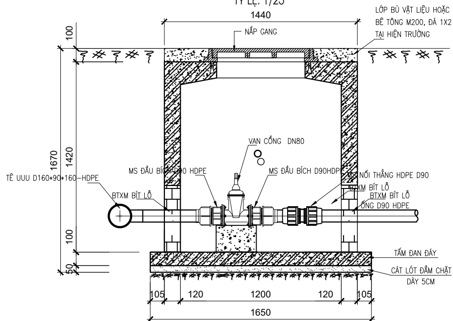
MẶT CẮT 1-1
