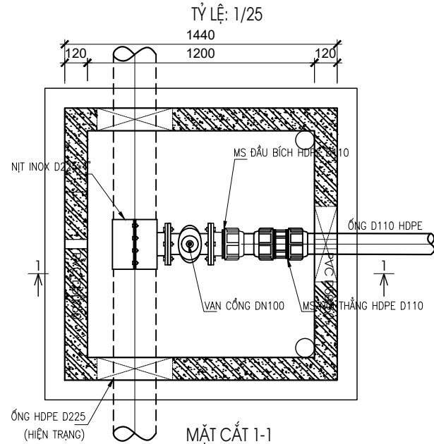
CHI TIẾT KHỞI THỦY ỐNG D110 HDPE VÀO ỐNG HDPE D225
