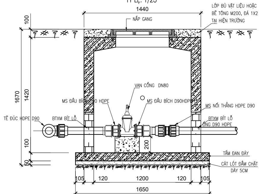
MẶT CẮT 1-1
