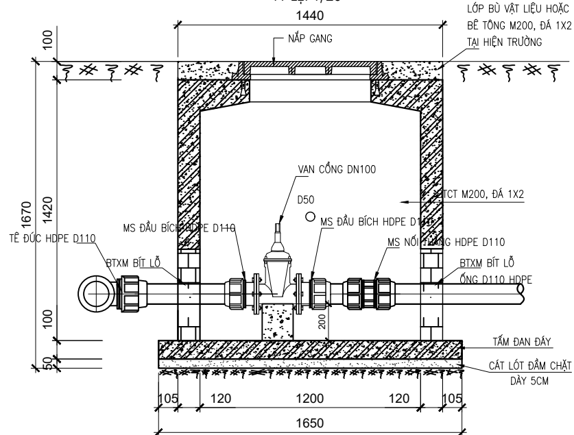
MẶT CẮT 1-1
