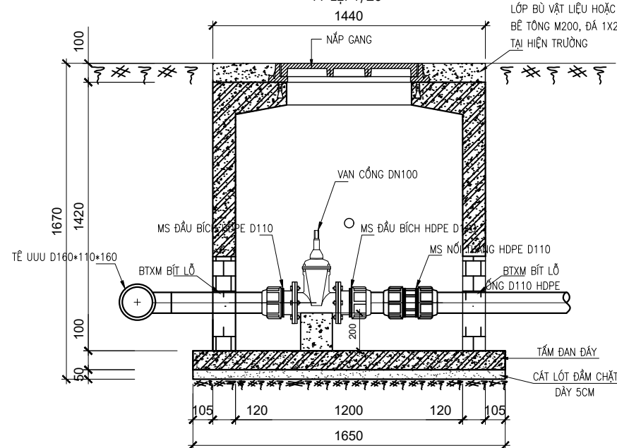
MẶT CẮT 1-1
