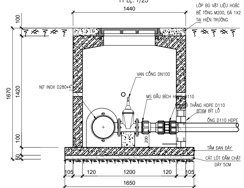
MẶT CẮT 1-1
