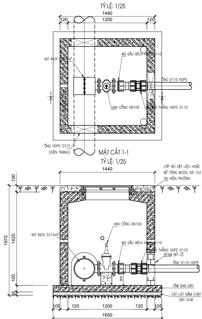
CHI TIẾT KHỞI THỦY ỐNG D110 HDPE VÀO ỐNG HDPE D315
