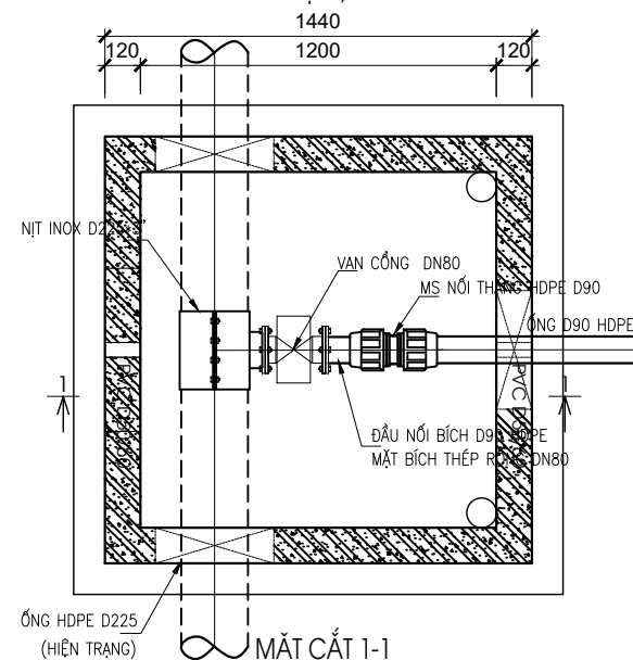
TỶ LỆ: 1/25
