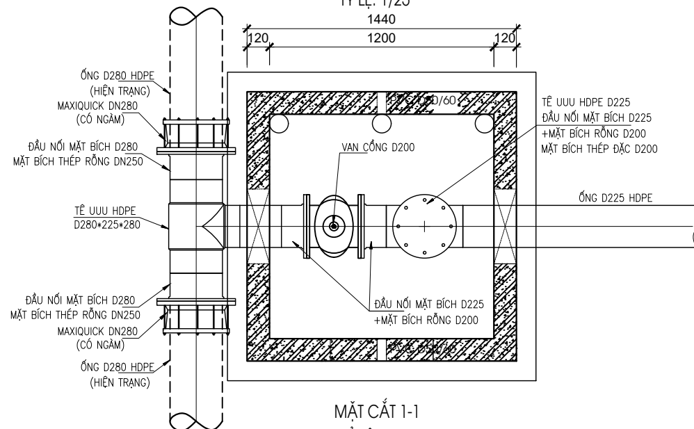
CHI TIẾT KHỞI THỦY ỐNG D225 HDPE VÀO ỐNG HDPE D280
