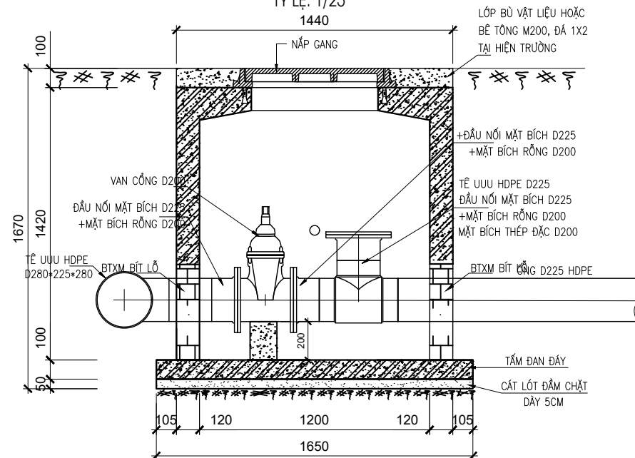
MẮT CẮT 1-1
