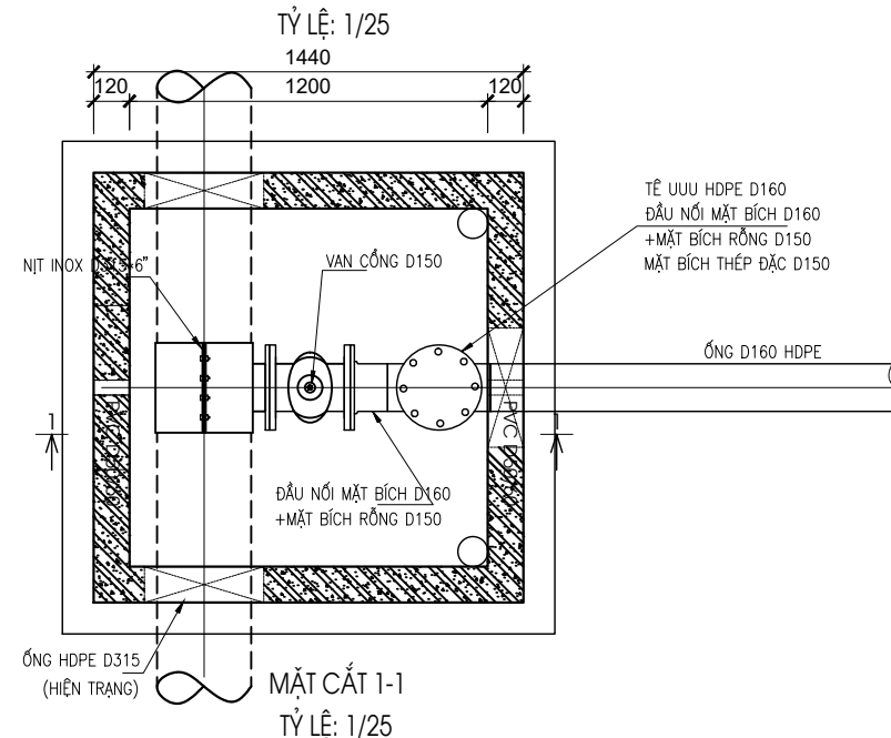
CHI TIẾT KHỞI THỦY ỐNG D160 HDPE VÀO ỐNG HDPE D315
