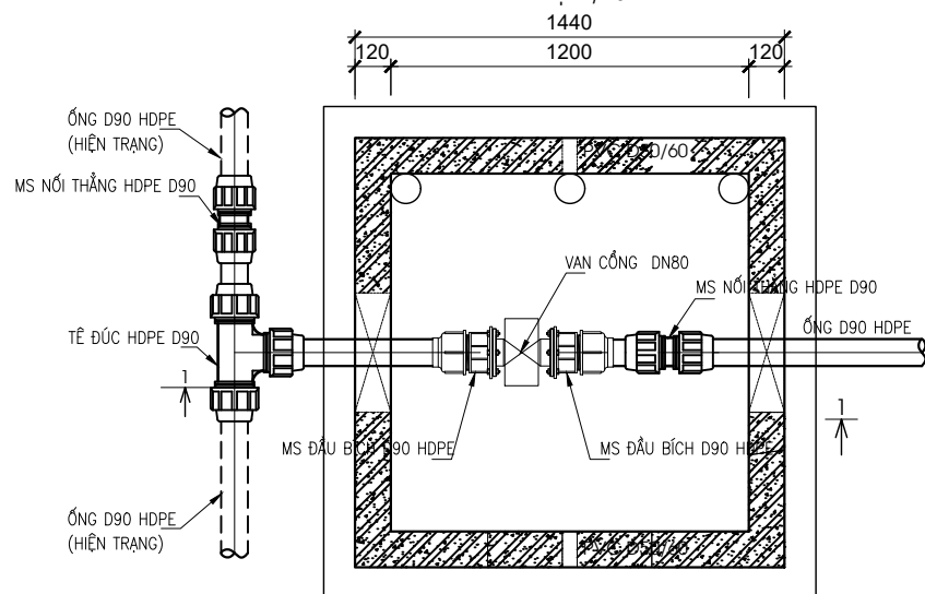
MẶT CẮT 1-1
