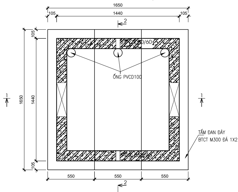
MẶT BẰNG HỐ VAN - TỶ LỆ: 1/25
