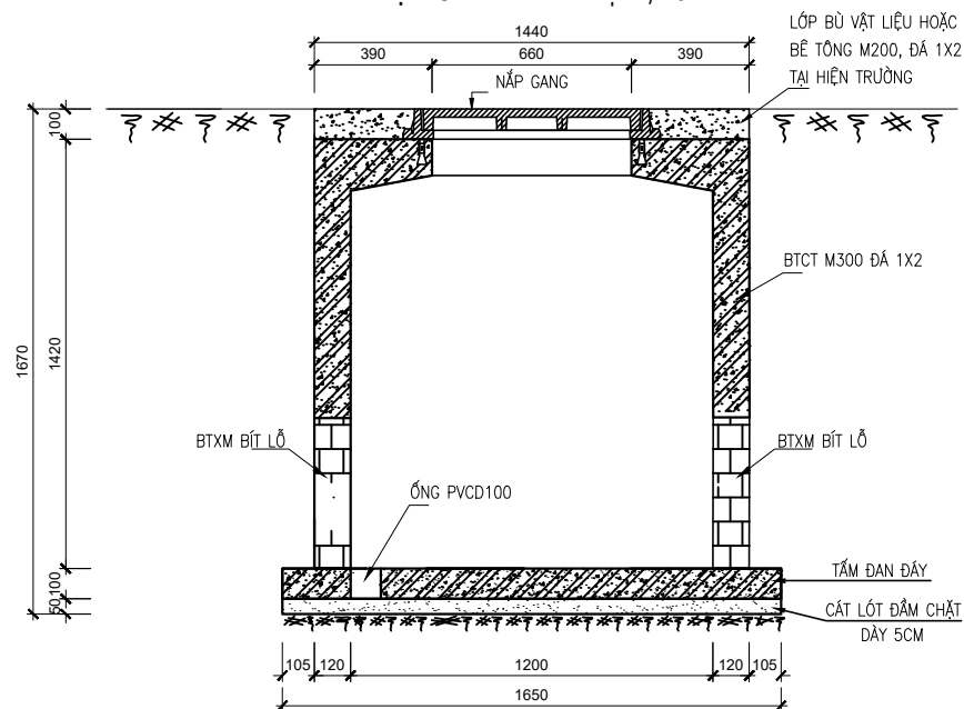
MẶT CẮT 2-2 - TỶ LỆ: 1/25
