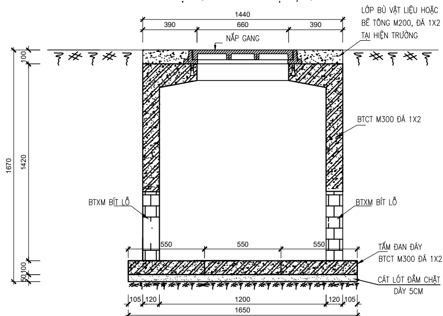
MẶT CẮT 1-1 - TỶ LỆ: 1/25
