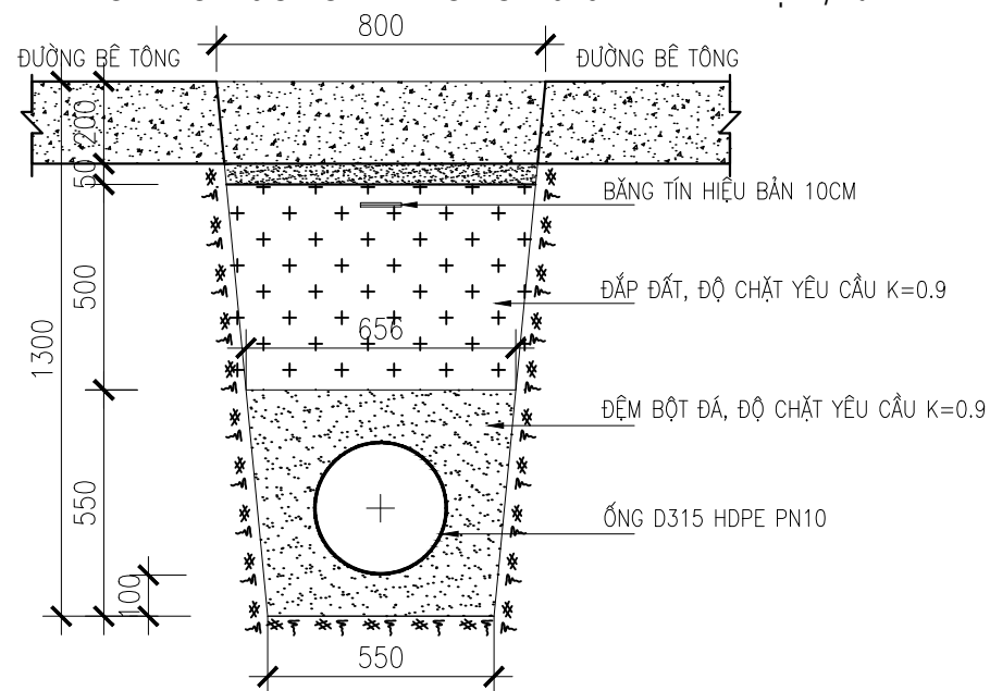
CHI TIẾT HỒ ĐÀO ĐƯỜNG BTXM ỐNG D315 HDPE - TỶ LỆ: 1/20
