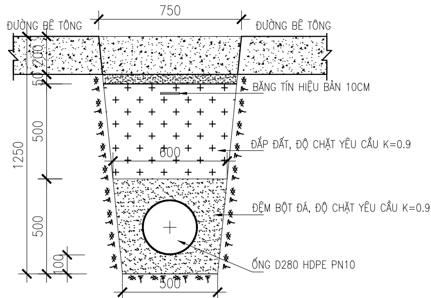
CHI TIẾT HỒ ĐÀO ĐƯỜNG BTXM ỐNG D280 HDPE -TỶ LỆ: 1/20
